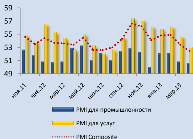
Индексы PMI
